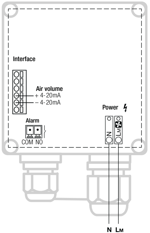
Input 4 - 20mA
